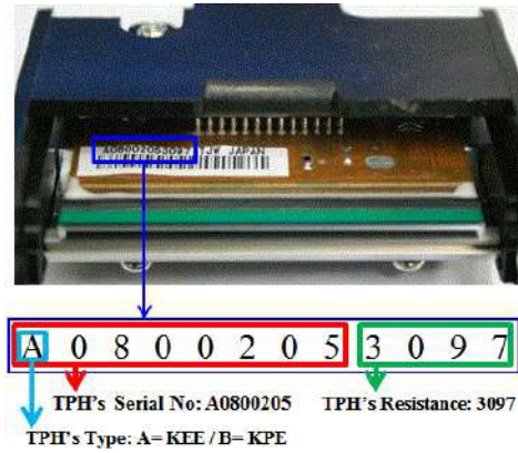
Рис. 111 Термопечатная головка
